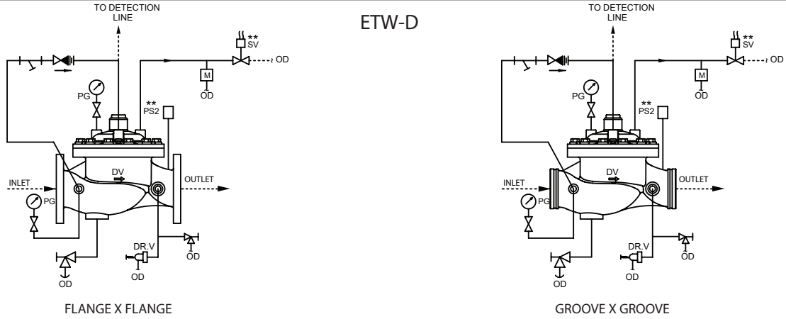
ETW-D SCHEMATIC 11
