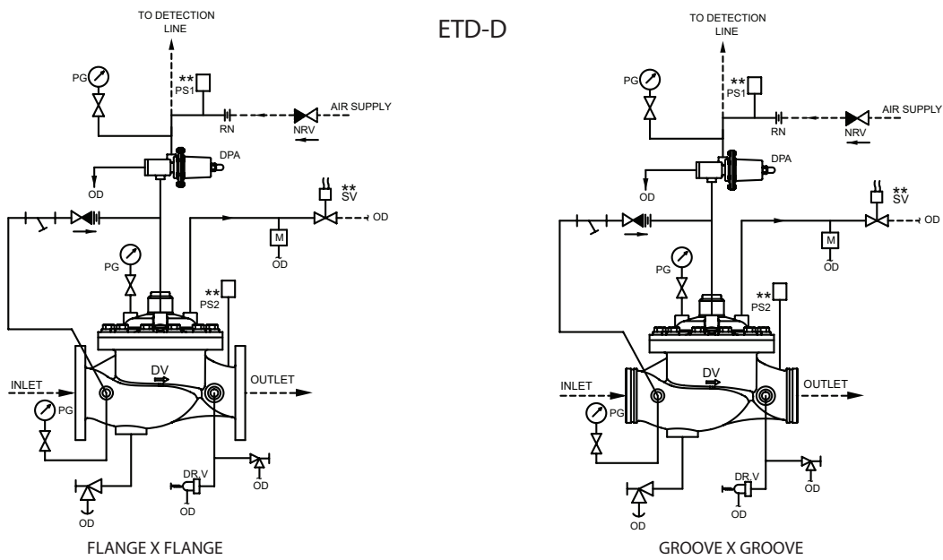
ETD-D SCHEMATIC 14
